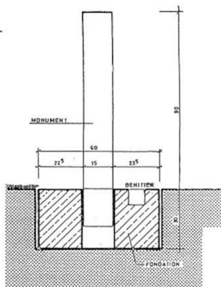
COUPE A-B 1/10
